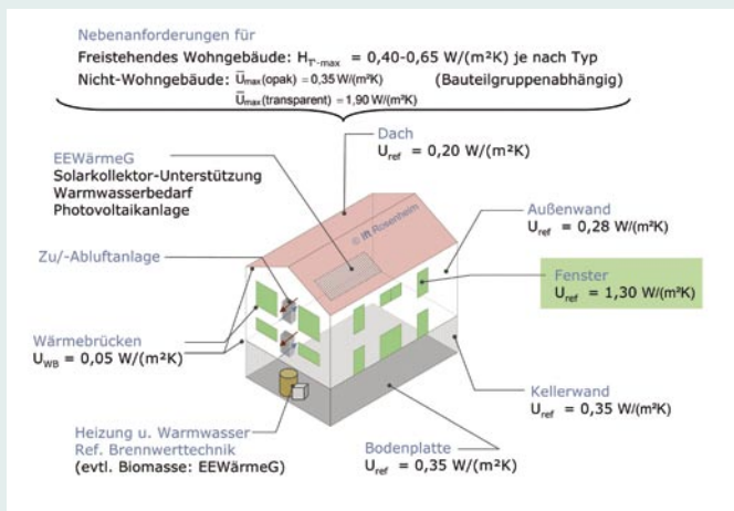
BILD 1: U-WERTE FÜR REFERENZGEBÄUDE IM NACHWEISVERFAHREN DER ENEV 2009
